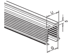
Guarnizione in gomma EPDM nera per tubo scanalato
